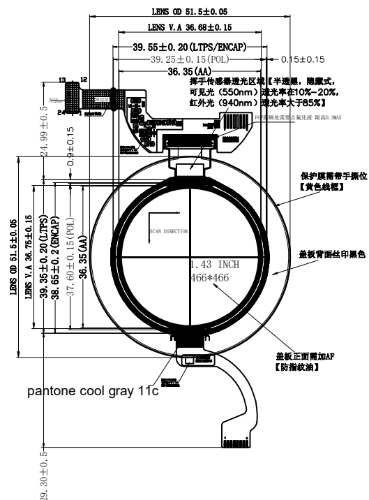
正视图
